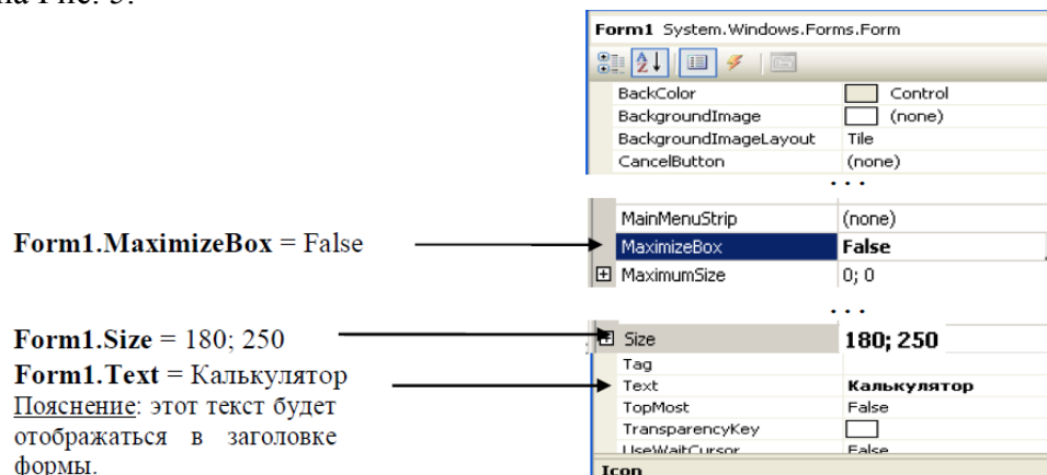
Рис. 5. Свойства Form1
