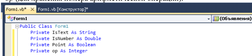
Рис. 6. Объявление переменных в блоке Form1 - Объявления
