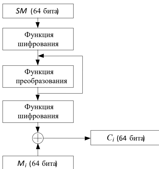
Рисунок 3. Работа алгоритма ГОСТ 28147-89 в режиме гаммирования с обратной связью Открытые данные T , которые подлежат шифровке, разбиваются на блоки T(j) длиной 64 бита.
