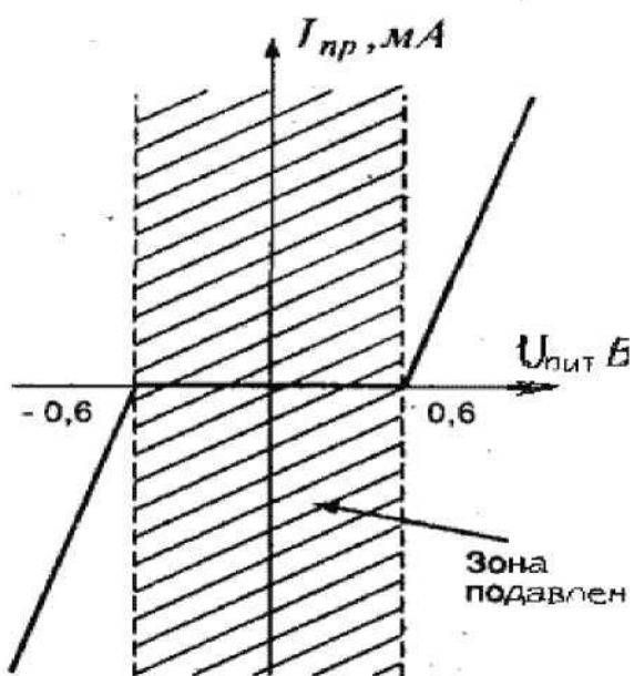
Рис. 1 .2. Вольтамперная характеристика диодов
