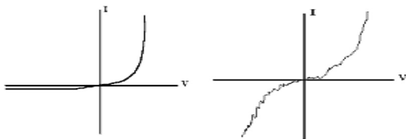
Рис.1. Вольт-амперные характеристики полупроводникового и ложного соединений. Из-за различия в нелинейных характеристиках полупроводникового и ложного соединений, отклики 2-й и 3-й гармоник будут иметь различную интенсивность. Когда НЛ облучает полупроводник, отклик на второй гармонике сильнее, чем на 3-ей. При облучении ложного соединения наблюдается обратный эффект: отклик на 3-ей гармонике сильнее, чем на 2-ой.
