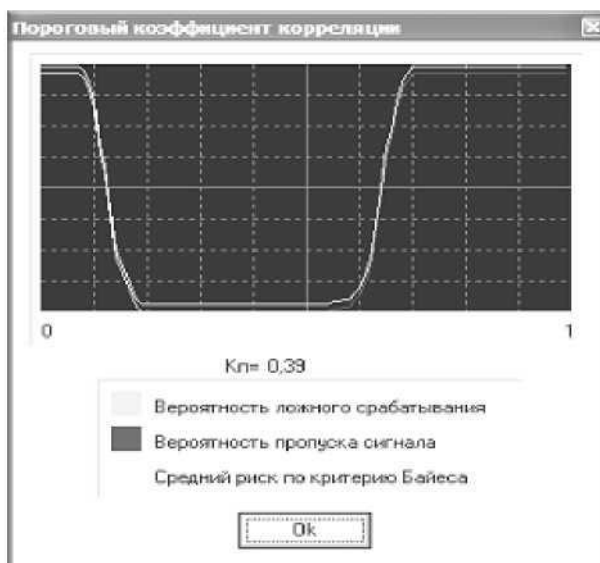
Рис. 2.6. Расчет порогового коэффициента корреляции
