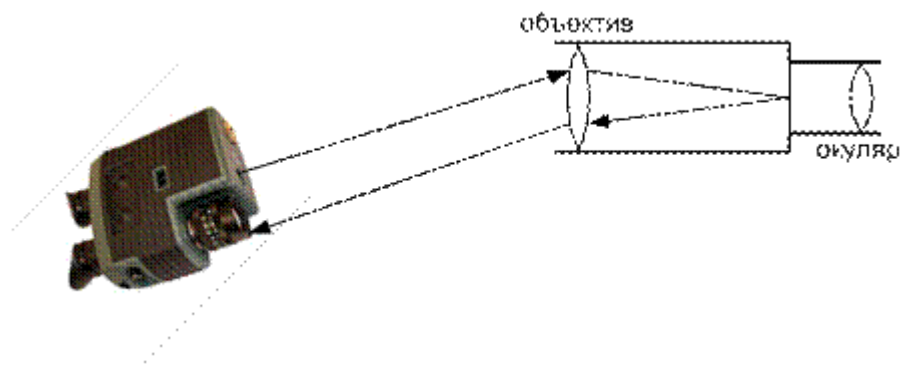
Рис. 2. Принцип действия обнаружителя оптических устройств
