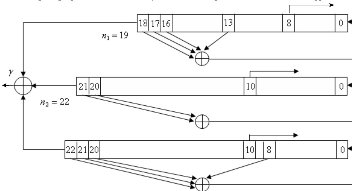
Рисунок 2. Алгоритм шифрования A5/1 стандарта GSM
