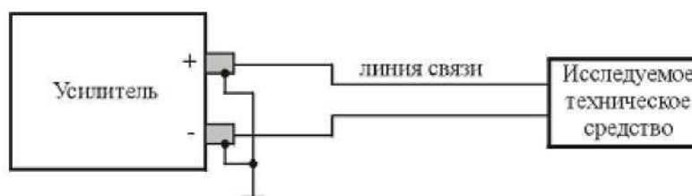
Рис. 1.4. Симметричная схема подключения
