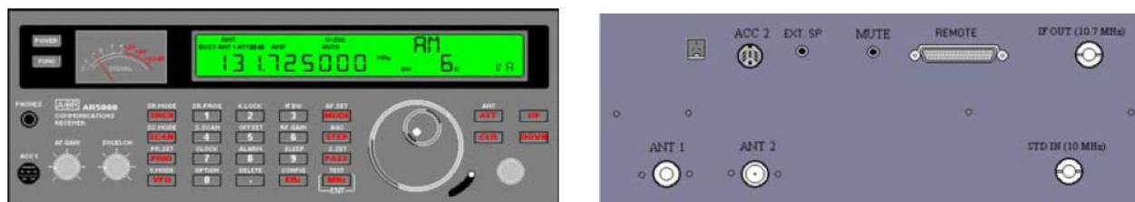
Рис.2 Передняя и задняя панель приемника
