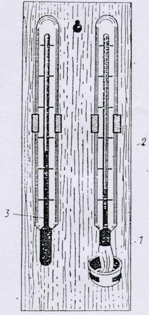
Рис. 2. Психрометр стационарный Августа:
