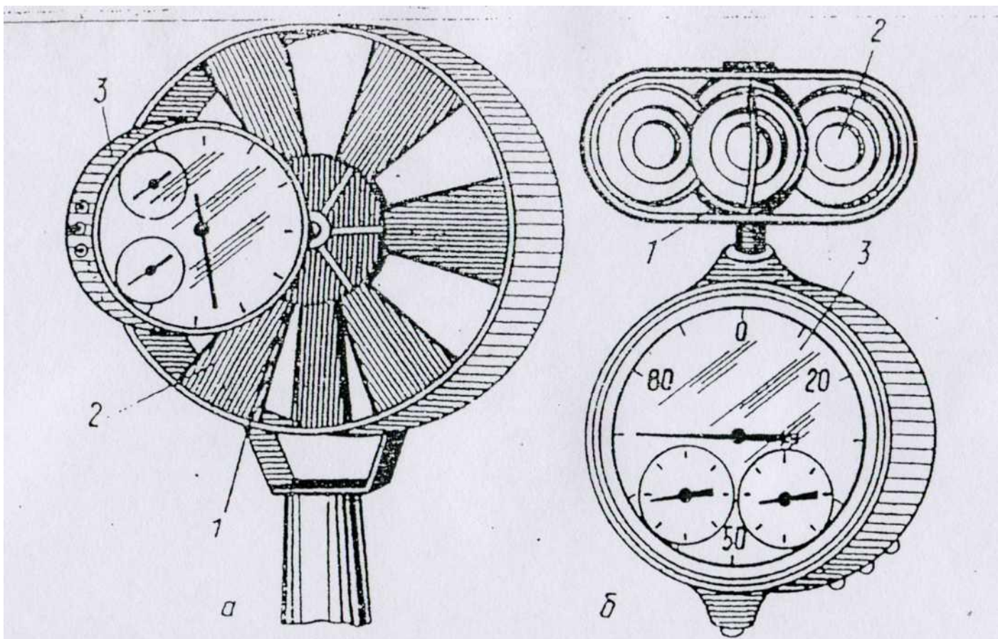
Рис. 5. Анемометры:
