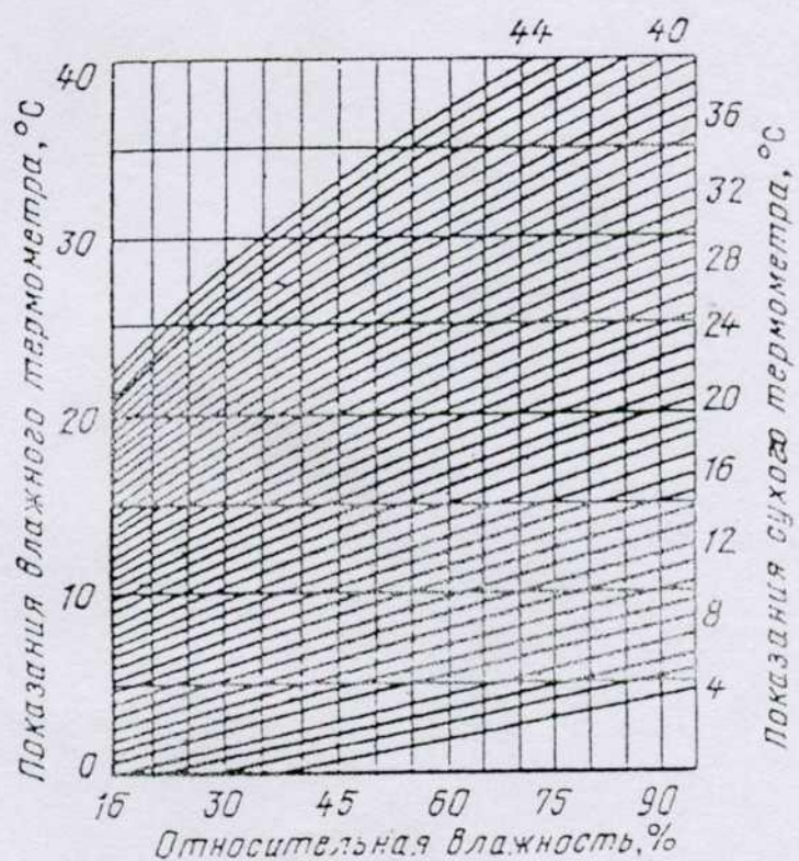
Рис. 4. Номограмма для определения относительной влажности воздуха по показаниям аспирационного психрометра
