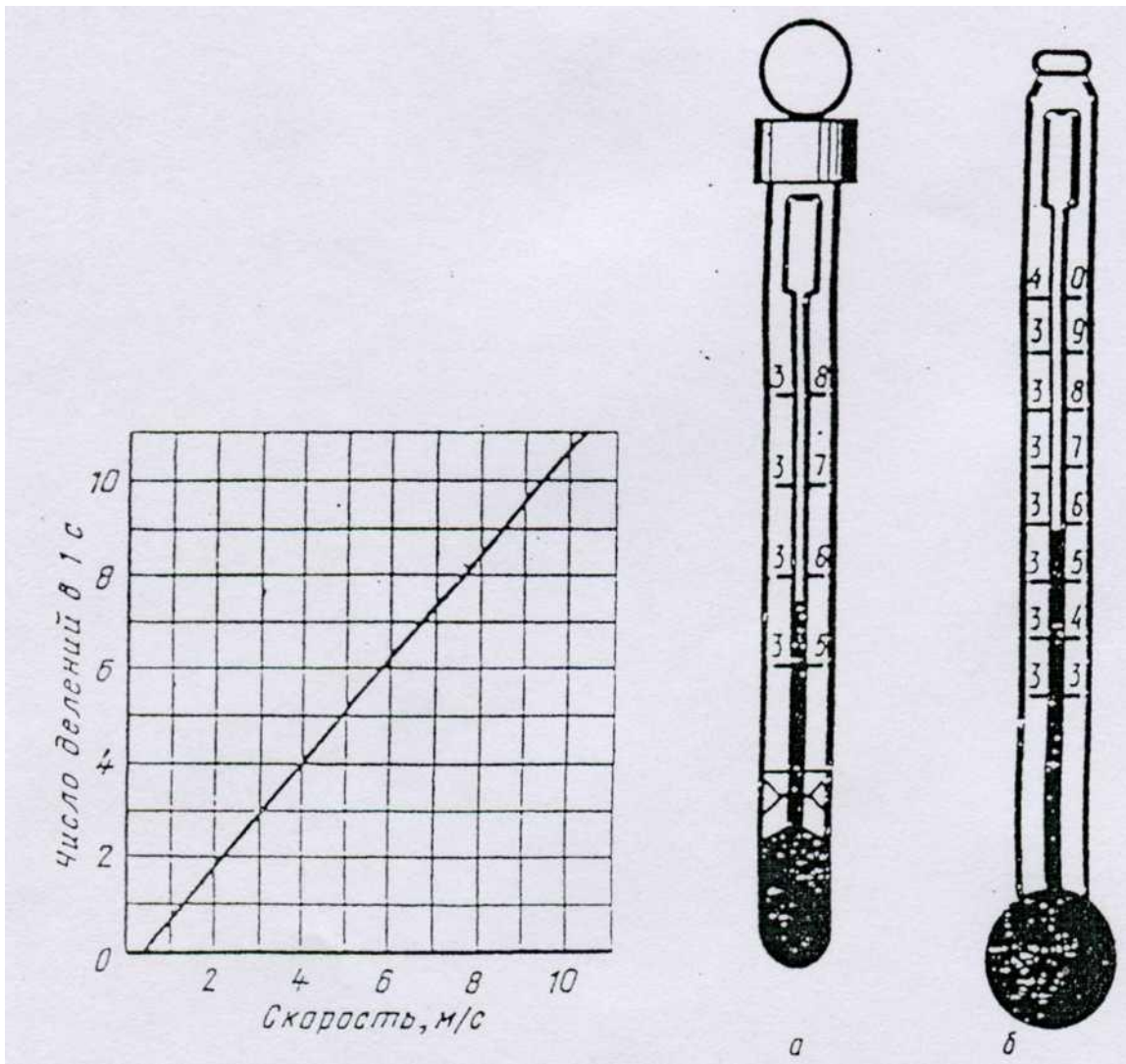
Рис. 6. График тарировочный ане- мометра.
