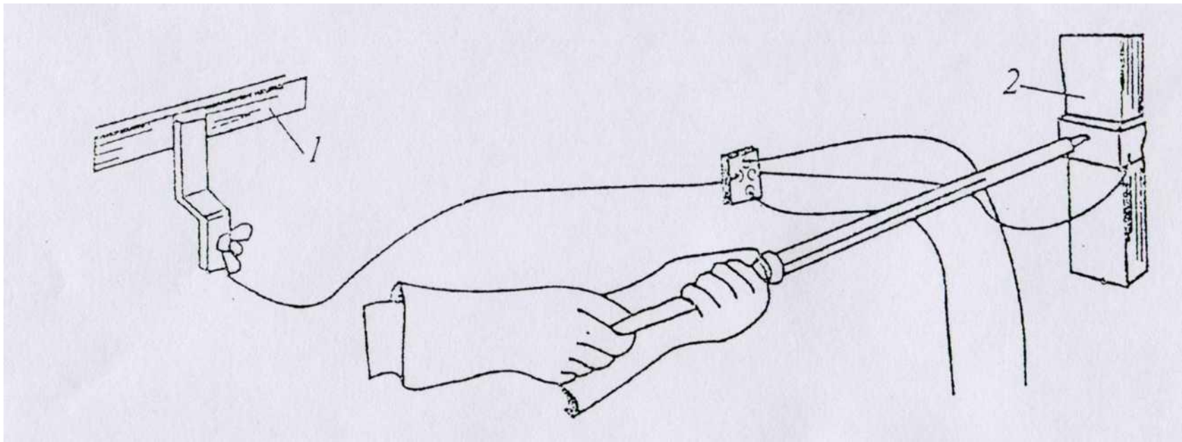
Временное переносное заземляющее устройство: / — шина сети заземления: 2 — токоведущая часть электроустановки
