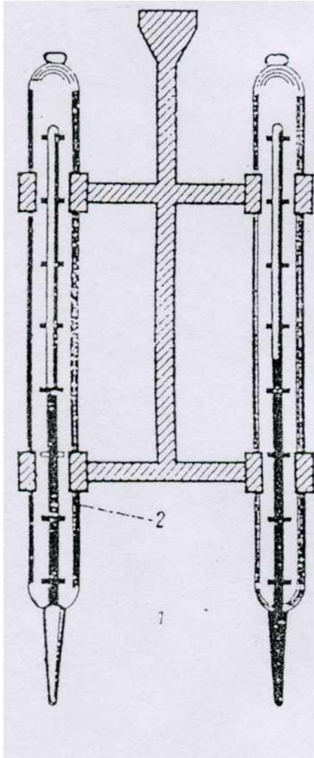
Рис. 1. Парный термометр
