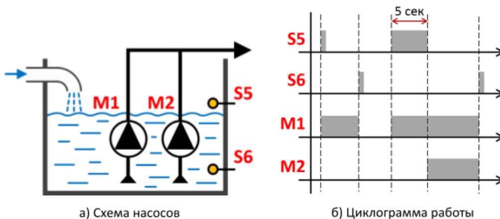
Рис.1 Насосная группа
