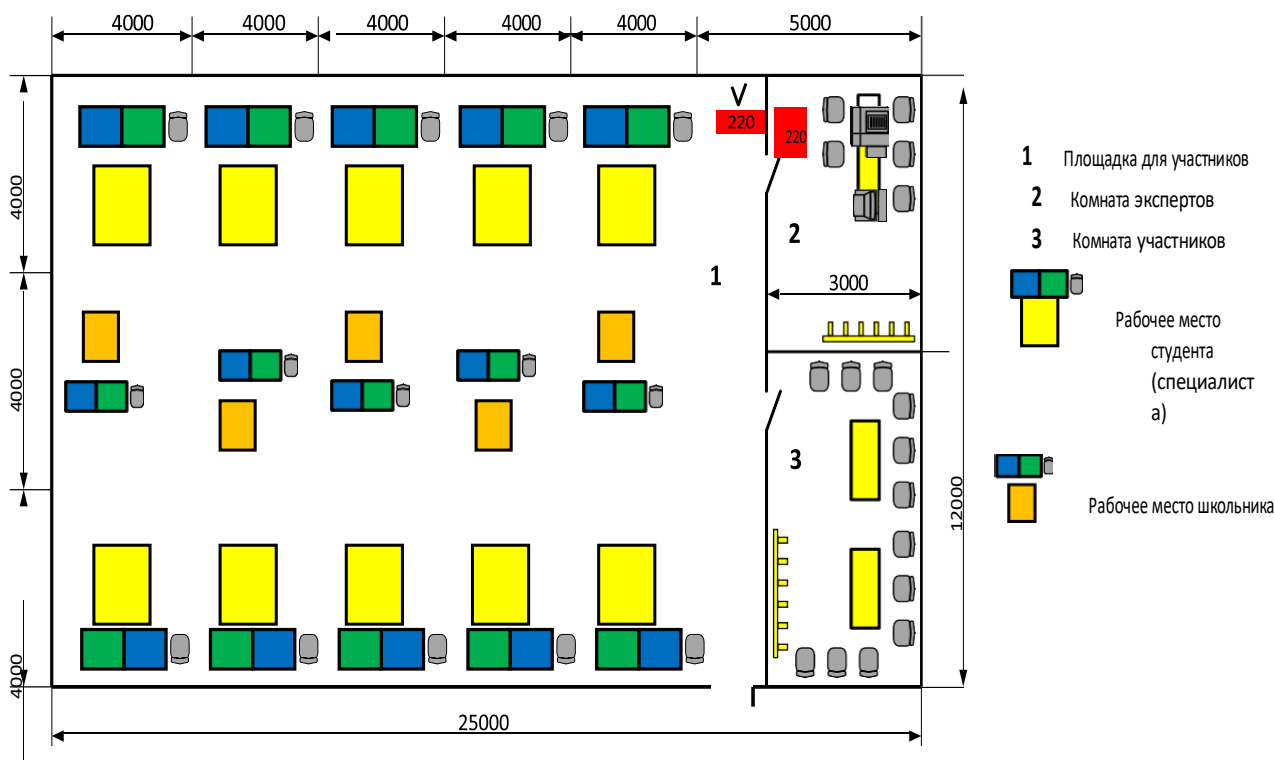
Рисунок 2 - Схемы застройки соревновательной площадки по компетенции – Ландшафтный дизайн
