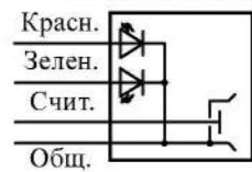
Считыватель Touch Memory
